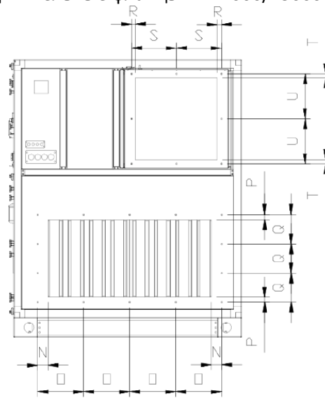
Соединительные фланцы AD11000/25000
