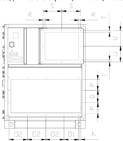
Соединительные фланцы AD7000/12000T
